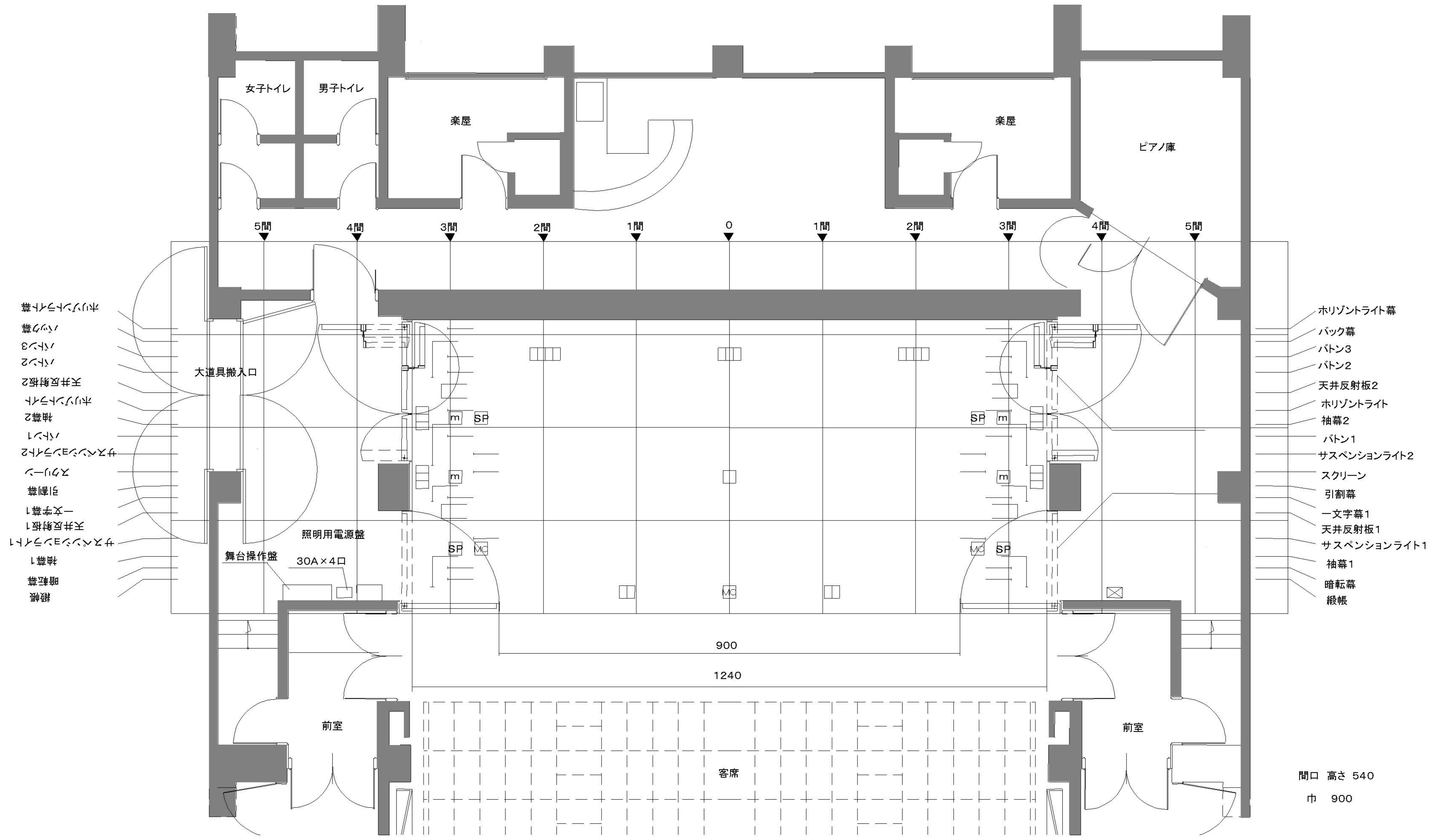
都の杜うぐいすホール 小ホール舞台平面図
